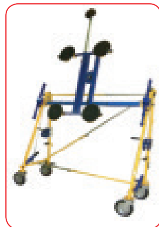
Nomad portata Kg 400 vetri max 4400 mm
