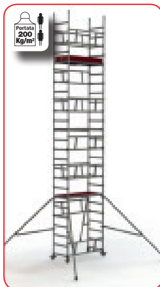
SVELTOWER montato alla massima altezza m 5,17
