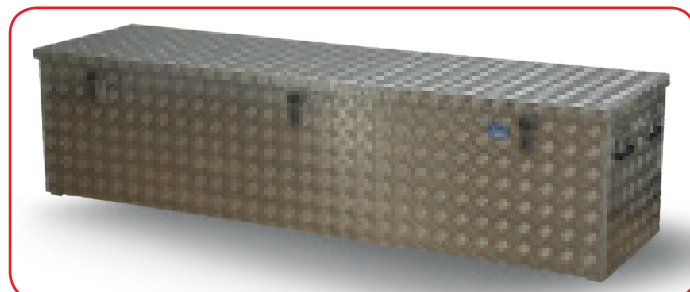
Serie Extreme (R) in alluminio mandorlato: uso pesante ed intensivo. Dotate di martinetti a gas di assistenza al sollevamento del coperchio. Presa per forche a richiesta.
