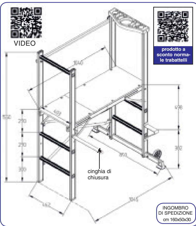
Portattrezzi integrato
