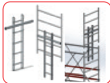
Servo System: nuovo accessorio per effettuare il montaggio in sicurezza delle spalle secondo EN1004.2
