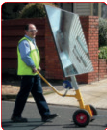
Express 150 - Peso tot Kg 92 (base Kg 30,6) (colonna Kg 44,6) (timone Kg 16,9)
