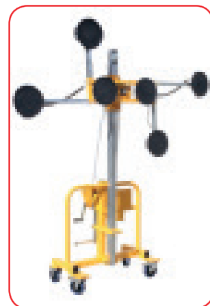
Mule portata Kg 300 vetri max 4400 mm
