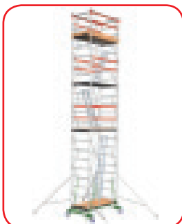
Professional EN1004 (completo di accessori)
