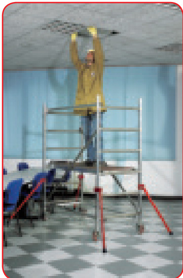
Millenium m 1,95 (Modulo A) con kit staffe S1 in acciaio obbligatorie per conformità alla EN1004.1.2
